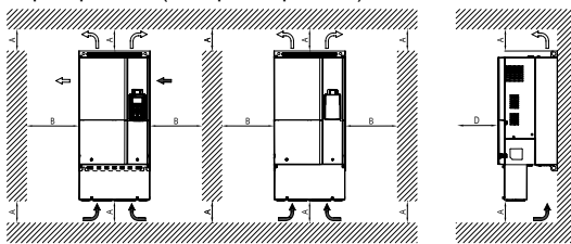
Рис. 4. Несколько ПЧ: Плотная установка (типоразмеры А-С)
